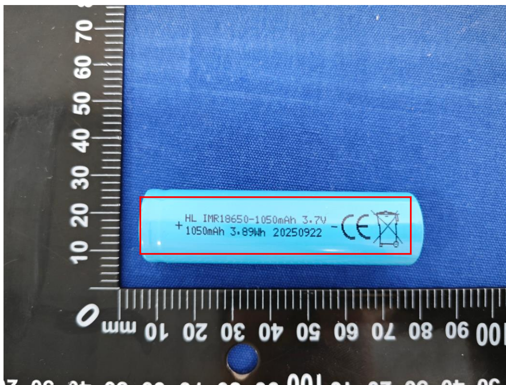
图七 产品外观（IMR18650-1050mAh）（红框为电池标签喷码位置）（标签样式二）
