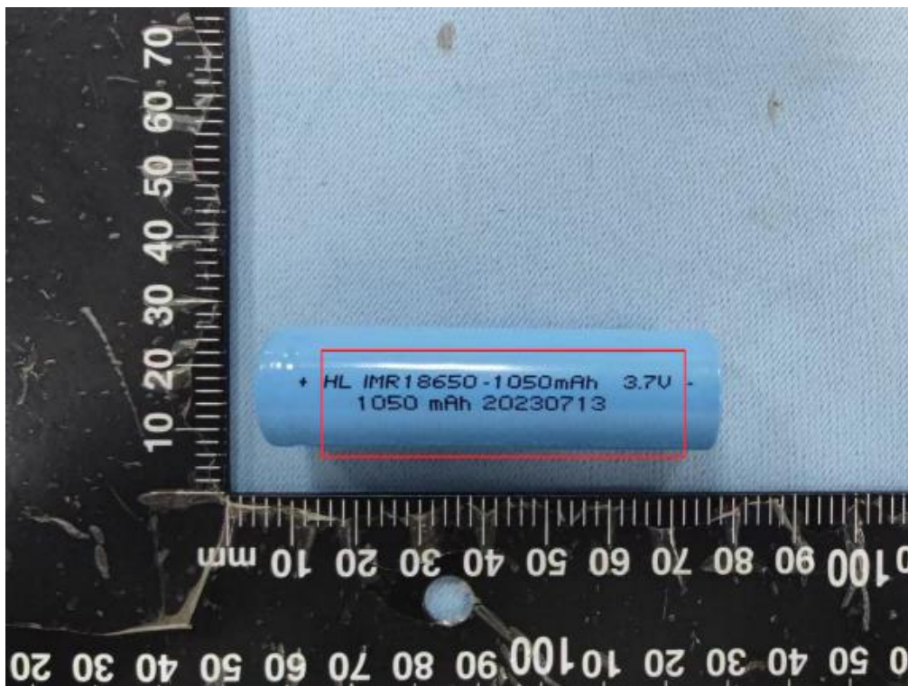
图五 产品外观（IMR18650-1050mAh）（红框为电池标签喷码位置）（标签样式一）
