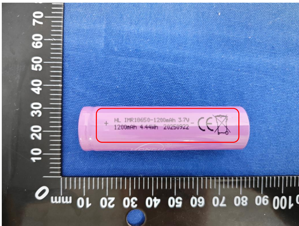
图三 产品外观（IMR18650-1200mAh）（红框为电池标签喷码位置）（标签样式二）
